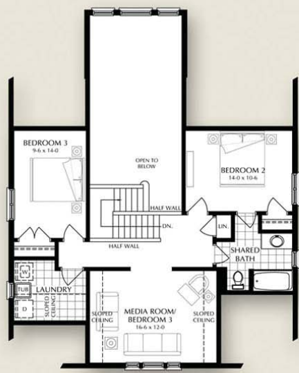
Optional Loft Floor Plan
